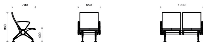
Model. SAIGA-01
